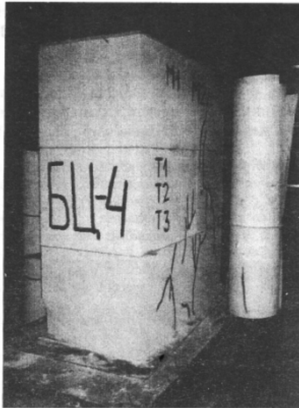
Рисунок 2 – Фрагмент кладки из газобетона марки по плотности D400 после испытания на центральное сжатие.
